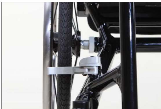
Abbildung 162: Anbringung der Integralbremse am unteren Rahmenrohr
