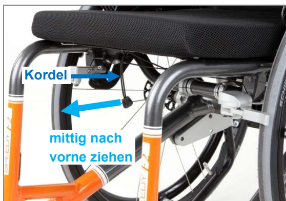
Abbildung 46: Kordel für die Betätigung der Rastbolzen
