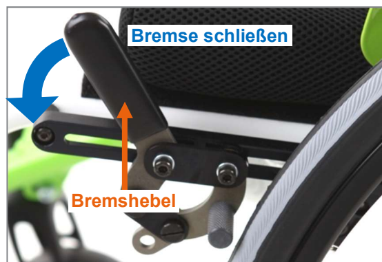
Abbildung 138: Bremse geöffnet; Schließen erfolgt durch nach vorne-unten Drücken des Bremshebels
