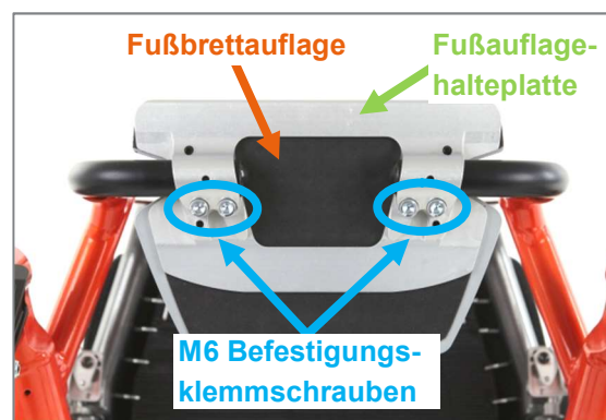
Abbildung 100: Fußstütze von unten
