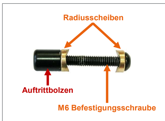
Abbildung 130: M6 Befestigungsschraube mit Radiusscheiben und Auftrittbolzen
