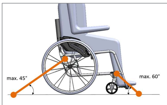
Abbildung 186: Verlauf der Retraktoren vorne und hinten mit maximalem Abspannwinkel und Anbindepunkten (Ansicht von der Seite)
